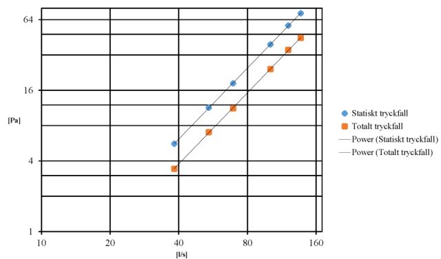
Tryckfallsdiagram uteluft vid vinkelrät montering
