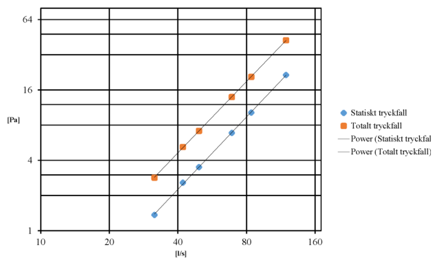
Tryckfallsdiagram avluft vid vinkelrät montering
